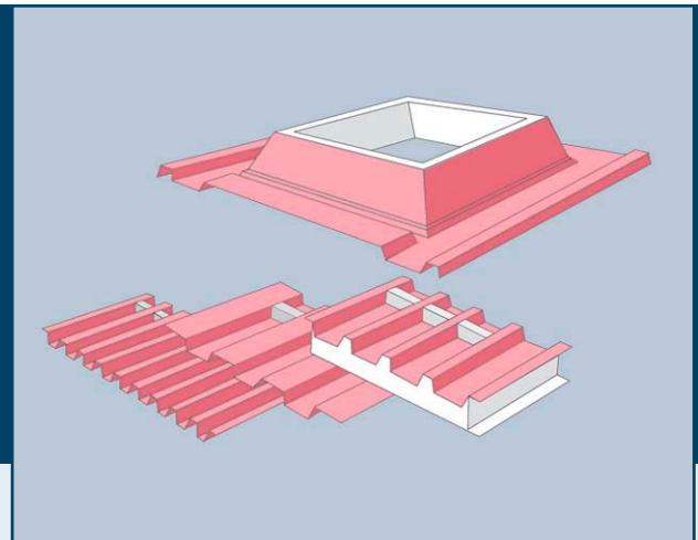
Teilprofilierte Ausführung
