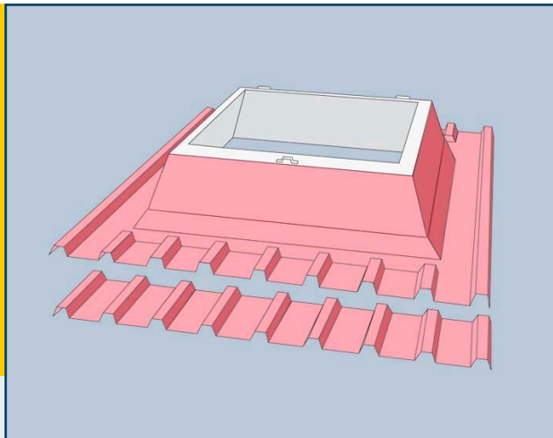
Vollprofilierte Ausführung
